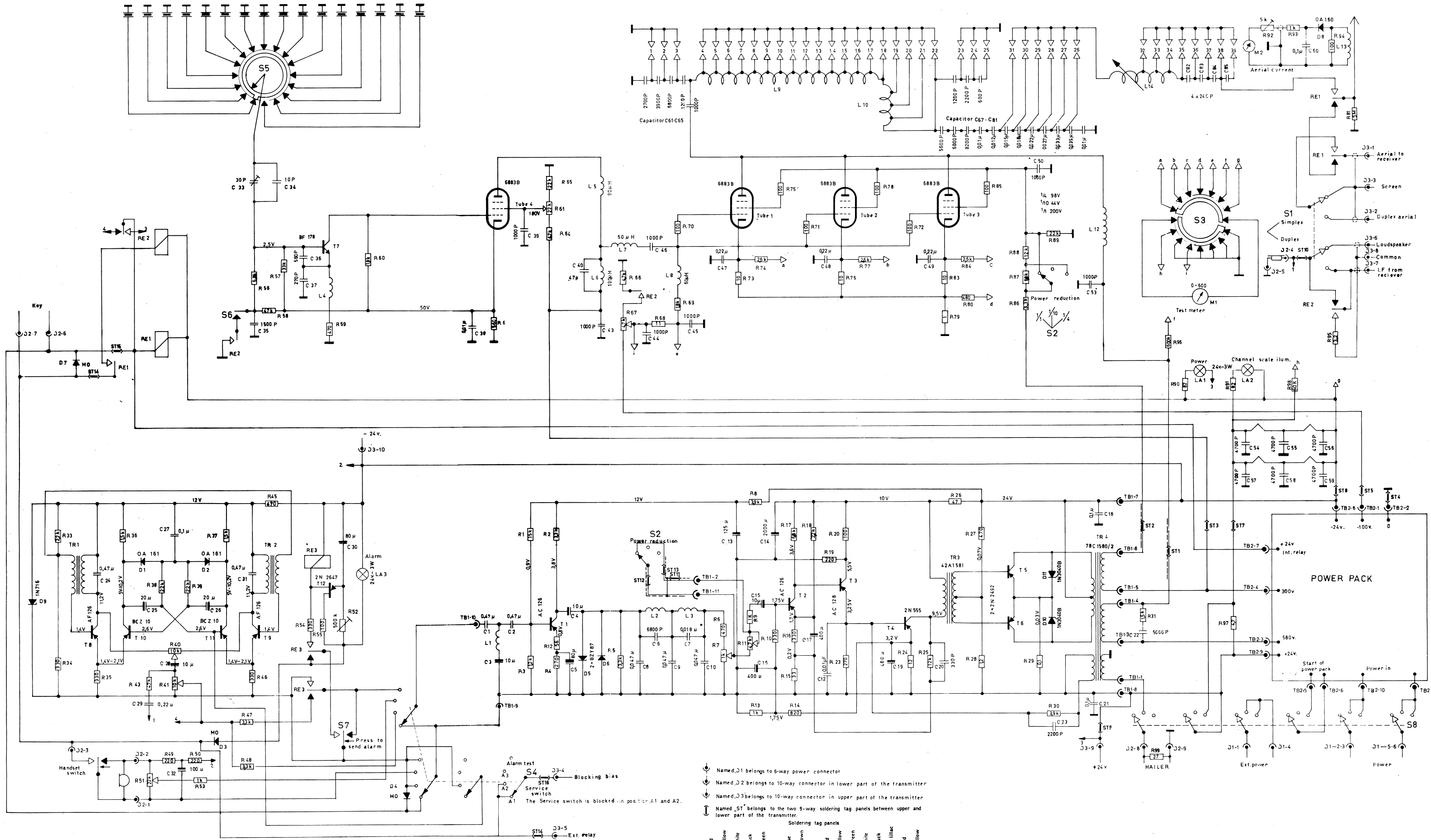
Dette skema omfatter SAILOR 56 D, serie D Dieses Schaltschema betrifft SAILOR 56 D, Serie D This diagram refers to SAILOR 56 D, series D Ce schéma s'étend au SAILOR 56 D, série D Este diagrama comprende SAILOR 56 D, serie D
