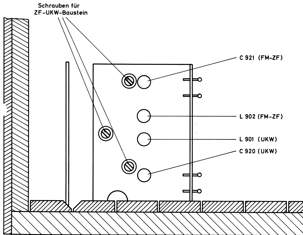
Abb. 8 Lage der Abgleichselemente für ZF- und UKW-Sender (Ansicht von oben)
