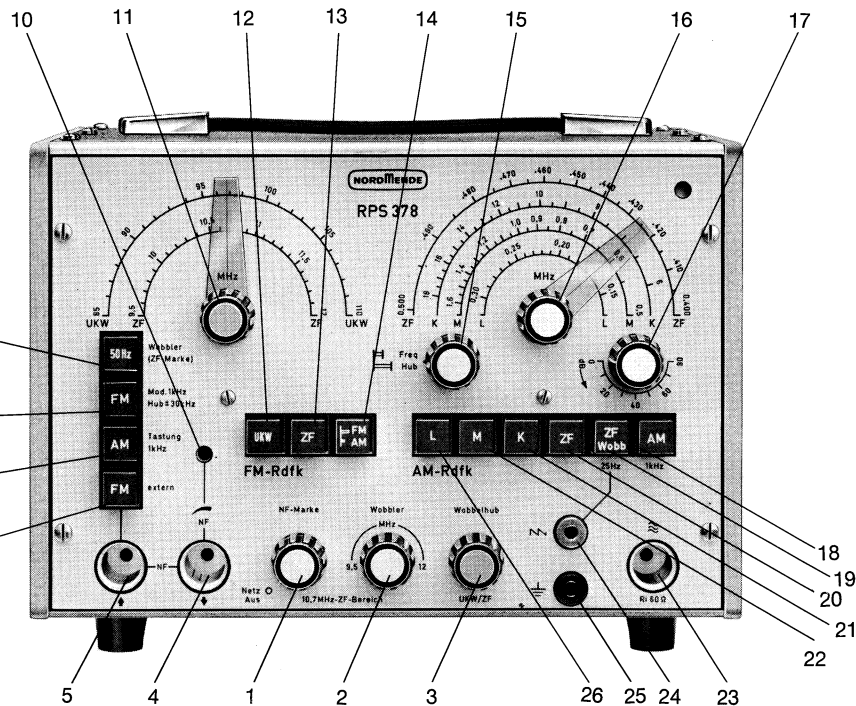
Abb. 2 Frontansicht
