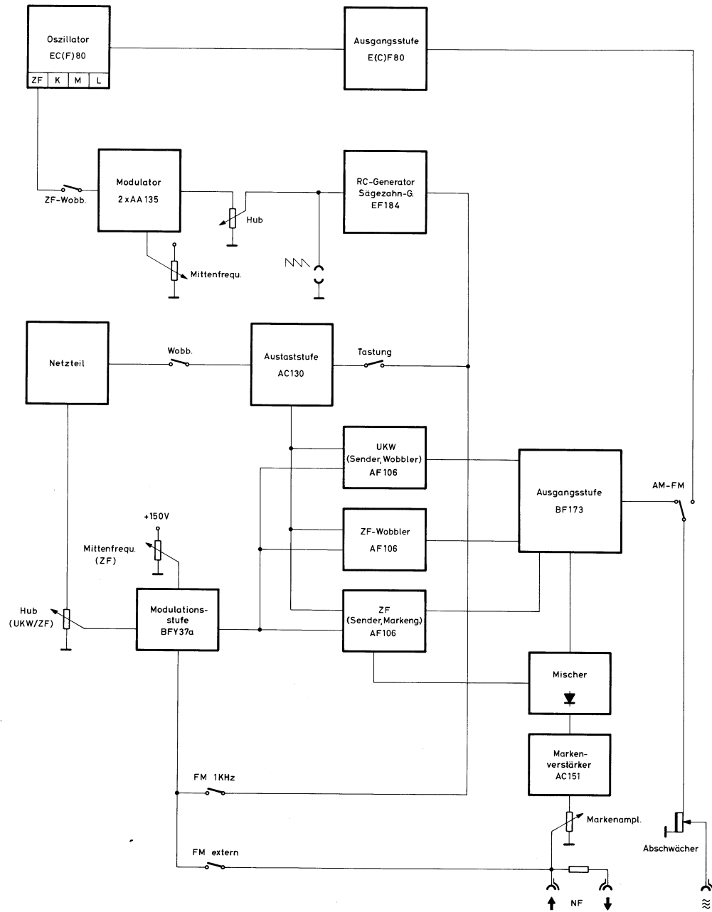
Abb. 5 Blockschaltbild RPS 378
