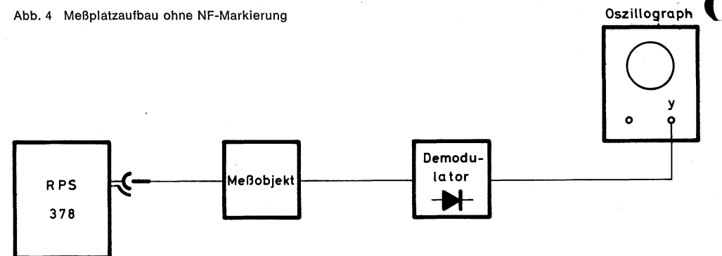
Abb. 4 Meßplatzaufbau ohne NF-Markierung
