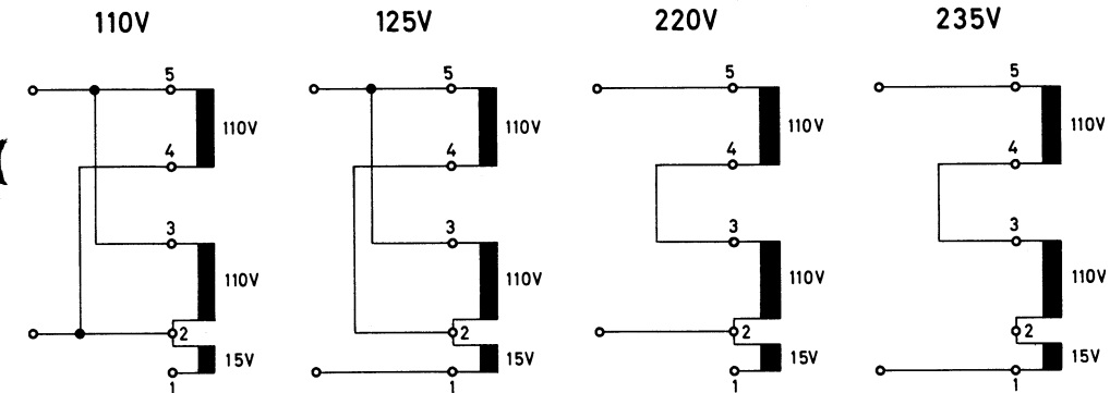
Abb. 1 Anschlußschema des Netztransformators
